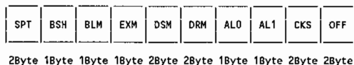
Bild 5-6: Der Disk-Parameter-Block
